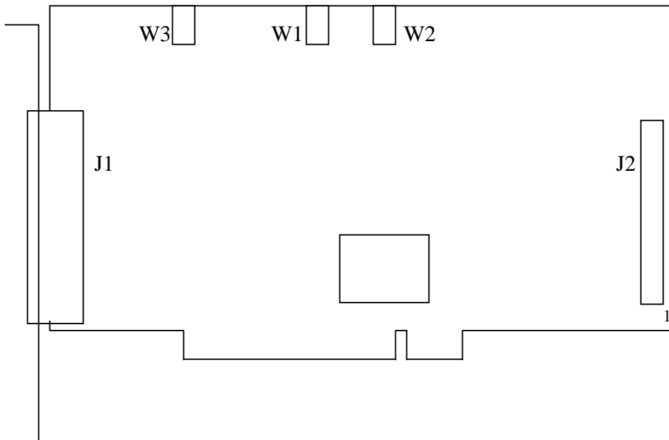
UA2011 卡布局图
