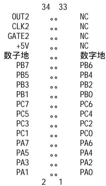
J2 数字信号连接座定义
